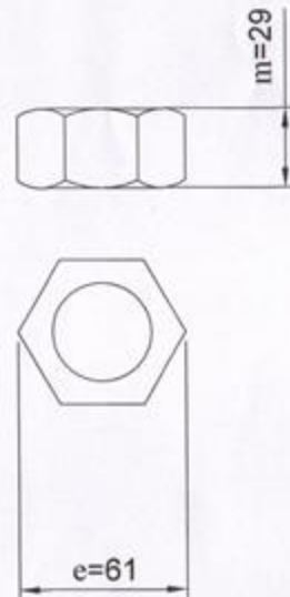
Part No.9 Nut M36 DIN 934
