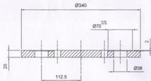
Sec. A-A
