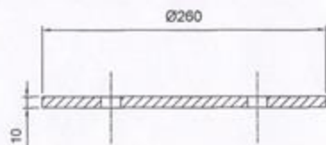
Sec. A-A
